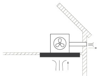
Motore installato sopra la cappa
